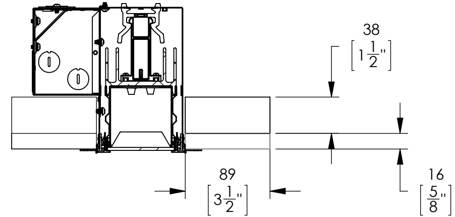
SECTION A-A FLANGELESS DRYWALL
